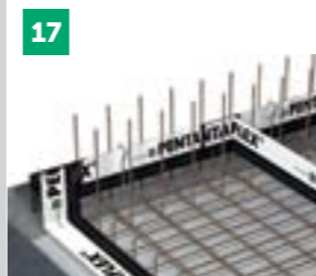
H-BAU PENTAFLEX® KB
